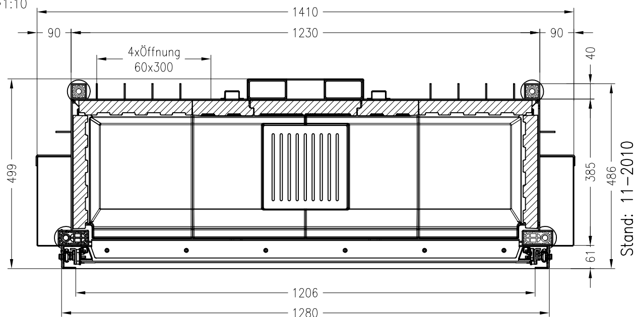
Horizontalschnitt M \approx 1:10
