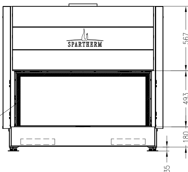
Vorderansicht M \approx 1:20
